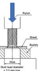
Ausdrückversuch
